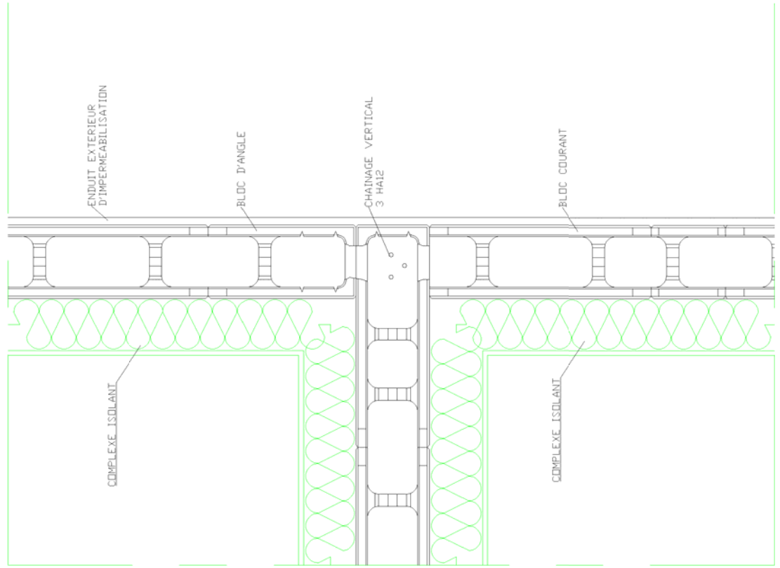
Figure 28a JUNCTION FACADE MUR DE REFEND EN MITOYENNETE BLOC ECLAIR TYPE 1
