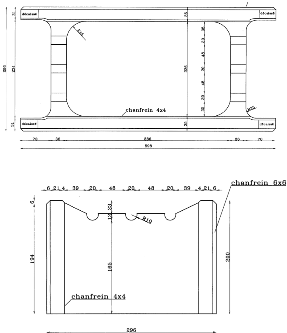
Figure 10 : bloc courant 600 x 300 x 200
