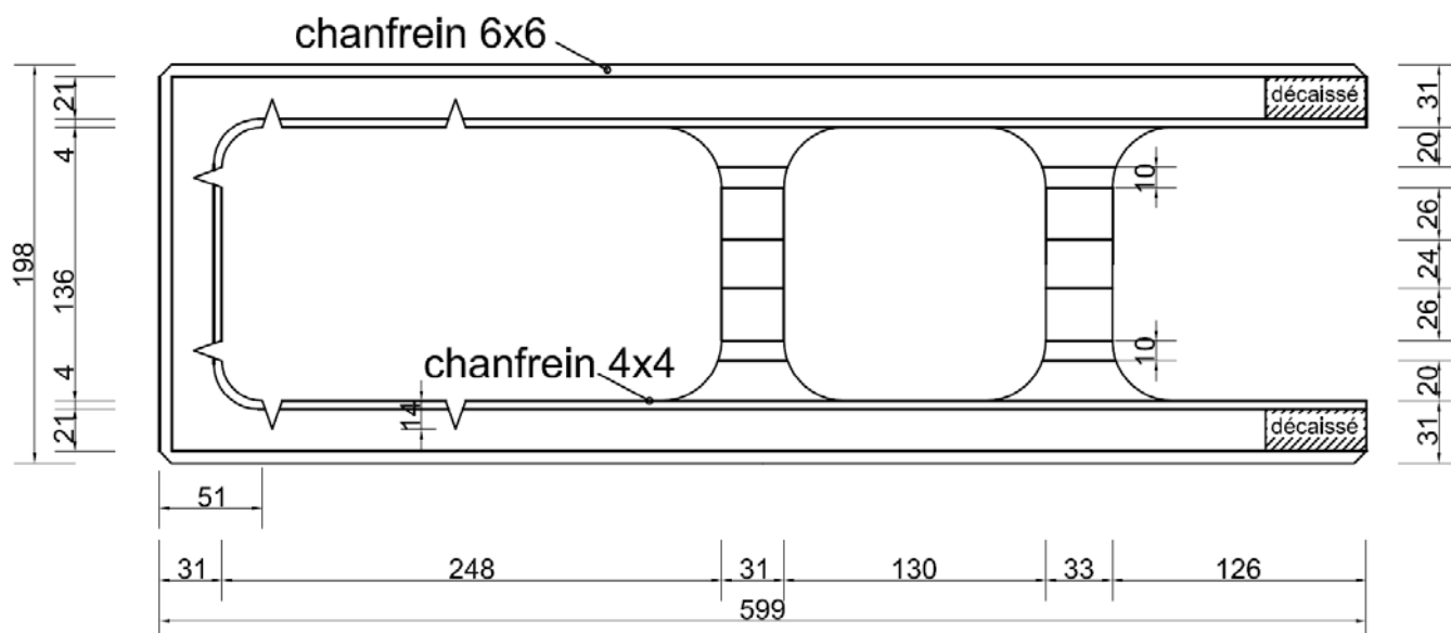
Figure 4 : bloc d'angle 600 x 200 x200
